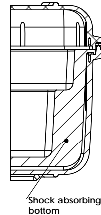
SECTION A-A
